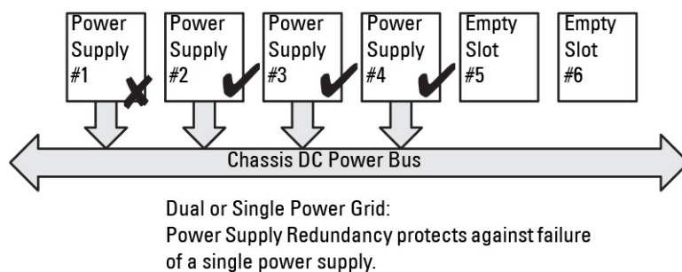
图 15: 电源设备冗余：合计 4 个 PSU，其中 1 个 PSU 故障
